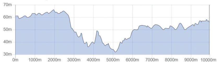
Profil trasy
